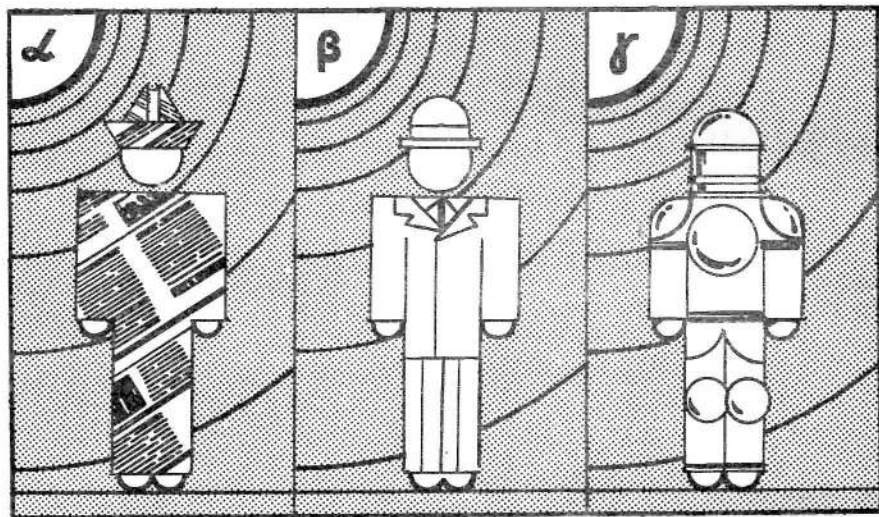
Рис. 1. Проникающая способность видов ионизирующего излучения различна: α-излучение можно затормозить тонким листом бумаги, β-излучение поглощается одеждой, γ-излучение ослабляется стенами домов, металлическими конструкциями
